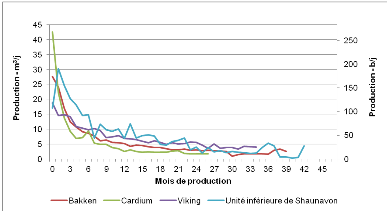
Figure 6 Profils de production des puits de pétrole de réservoirs étanches
