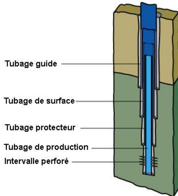
Figure 8 Structure typique d'un puits
