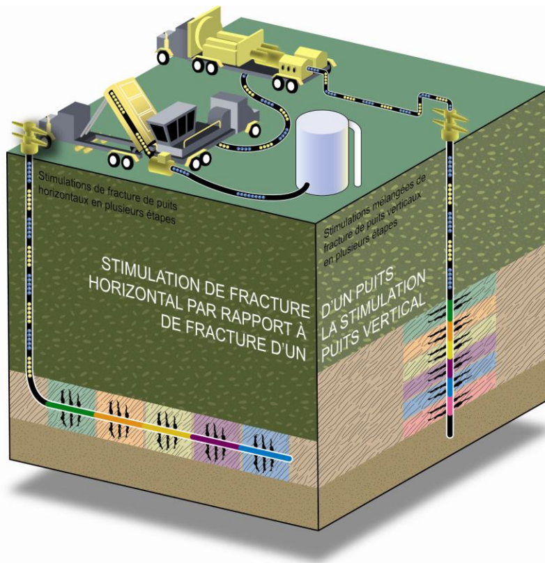
Figure 9 Fracturation hydraulique en plusieurs étapes dans les puits horizontaux et verticaux
